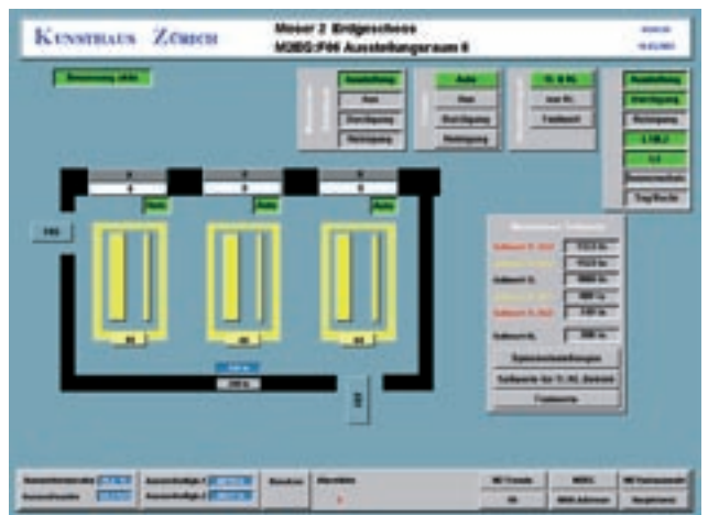
Über das GA-Leitsystem Saia®ViSi-PLUS werden die Sollwerte für jede Ausstellungszone getrennt eingegeben und überwacht.
