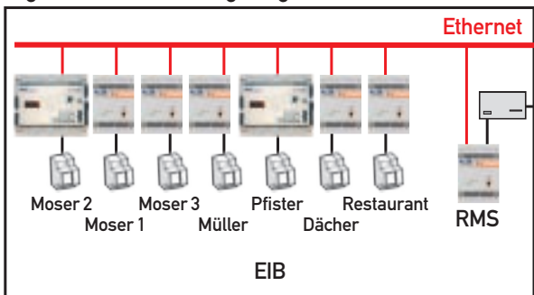
Kommunikationsschema zu den HLKS-Anlagen und der Lichtregelung
